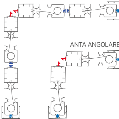
2 ANTE A SEGUIRE ANGOLARE
