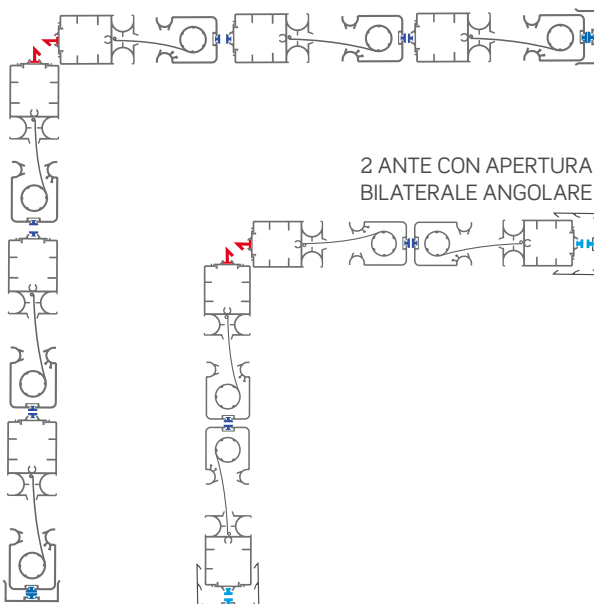
3 ANTE A SEGUIRE ANGOLARE
