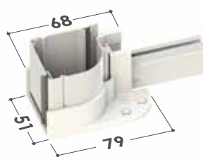
Cassonetto da 45 Testate inferiori
