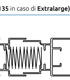
Profilo portarete
