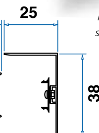
Profilo di compensazione per grandi fuorisquadro. (opzionale)
