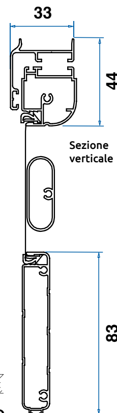
Profilo fascia inferiore
