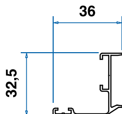
Profilo telaio
