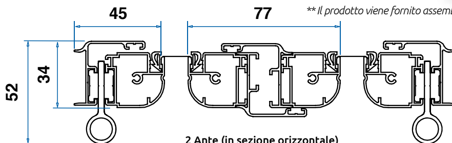
2 Ante (in sezione orizzontale)
