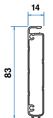
Profilo fascia inferiore
